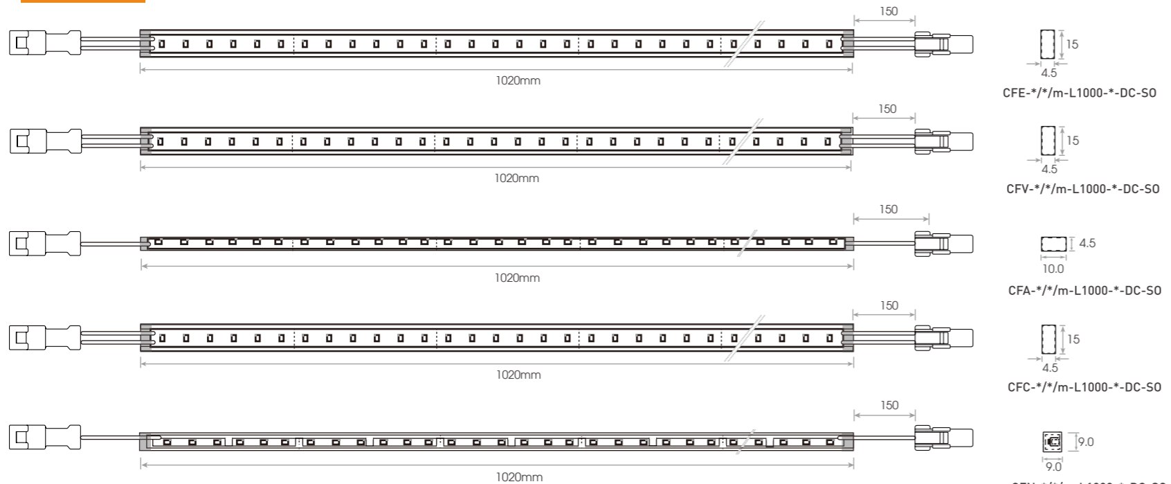
*L1000双端直出线标准品图 *所有系列均可做单端出线
