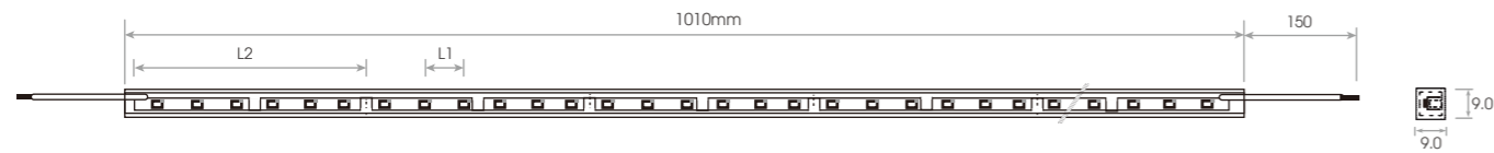
*L1000双端直出线标准品图
