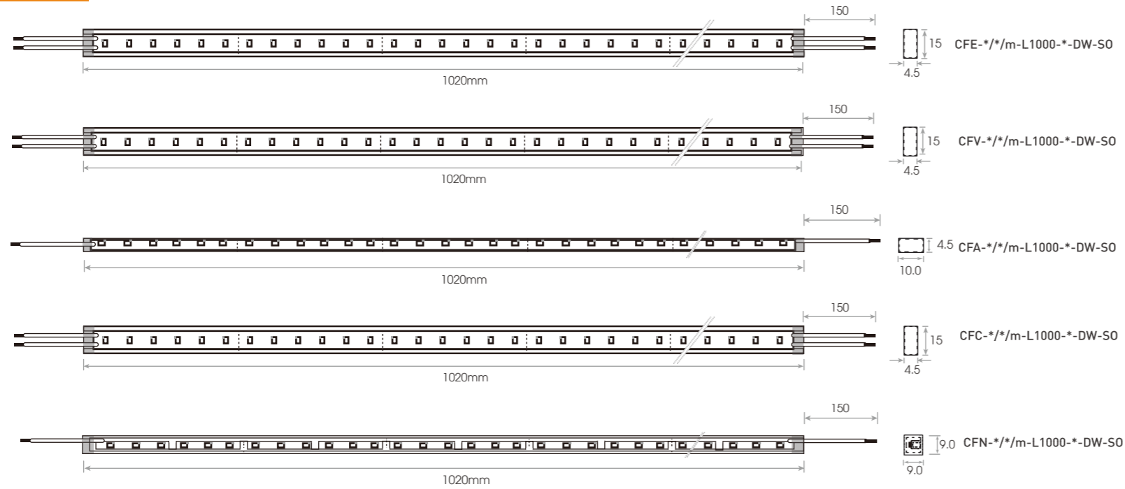
*L1000双端直出线标准品图 *所有系列均可做单端出线
